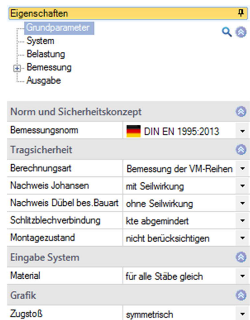
Abb: HO3+
