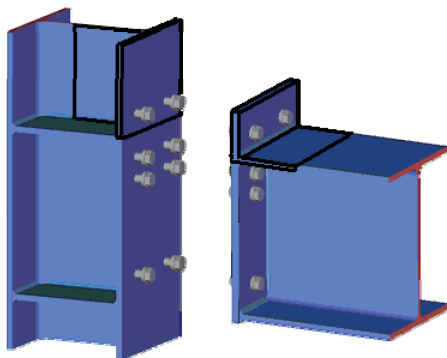
Bsp. T-Stummel in ausgesteifter Stütze Teil 1 Teil 2
