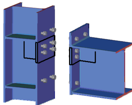
Bsp. T-Stummel in ausgesteifter Stütze
