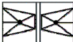
nicht kreisförmige Muster l_{eff,nc}
