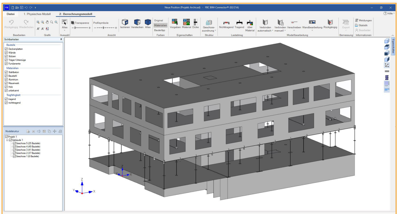
Abb. 16: Das Berechnungsmodell
