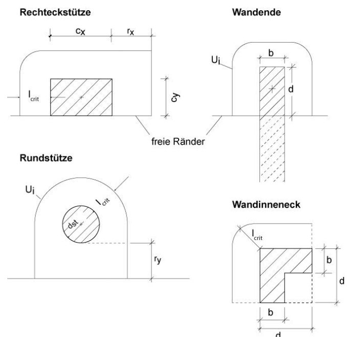
Abb. 1: Kritischer Querschnitt bei Rand- und Eckstütze, Wandende und -innenecke im Abstand
