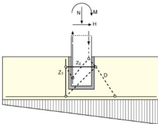
Abb. : Ermittlung der lotrechten Bügel As_v mit Zugkraft Z_1 , Ermittlung der horizontalen Bügel As_h mit Zugkraft Z_2
