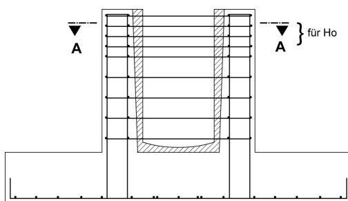
Schnitt A-A
