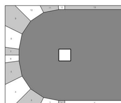
Randstütze
