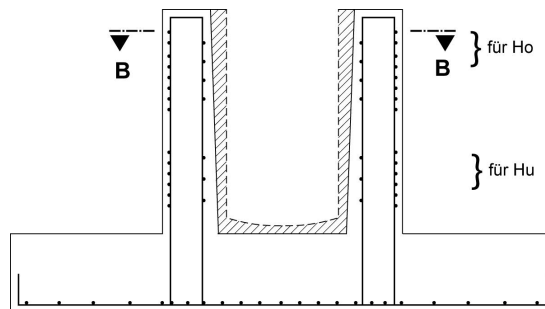
Schnitt B-B
