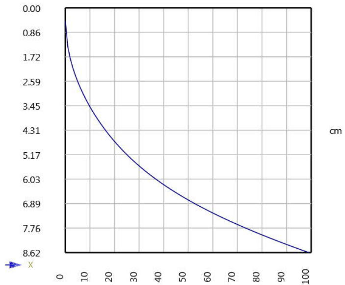
Zeitsetzungsverlauf bis zum geschätzten Abschluß der Konsolidation in Tagen und cm
